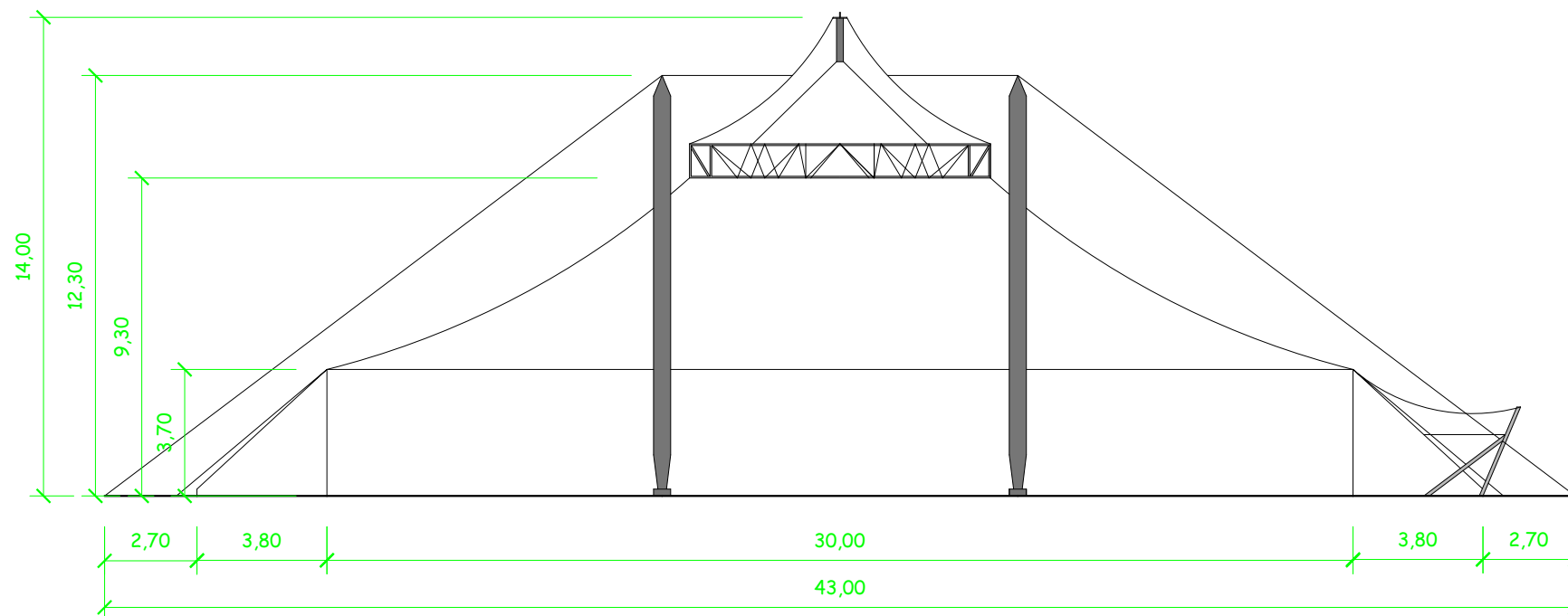
Coupe AA
